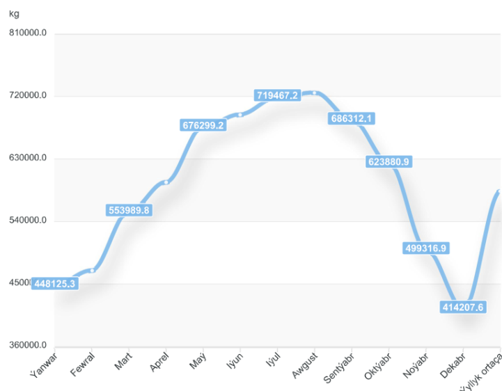
Рис. 1. Количество сэкономленного количества природного газа при использовании электролизеров для получения 885 кг водорода
