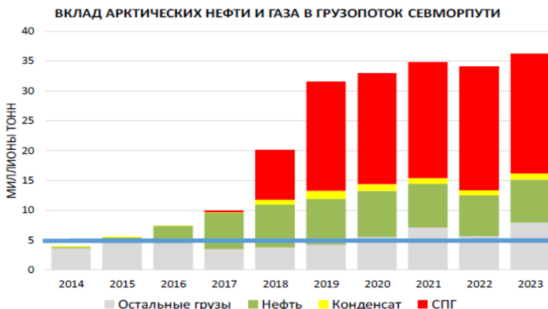
Рис. 2. Объем грузопотока арктической нефти, конденсата и СПГ
