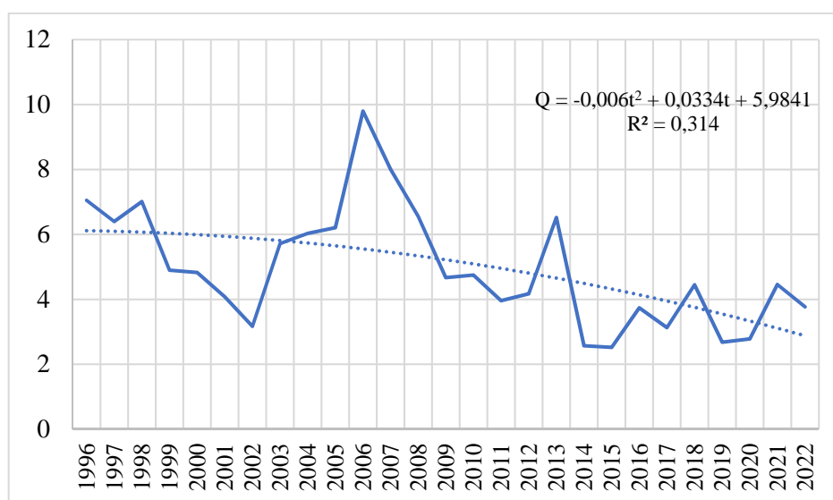
Рис. 3. Среднегодовые расходы воды (Q, м 3 /с) р. Ворсклы (пост Козинка) за 1996–2022 гг.
