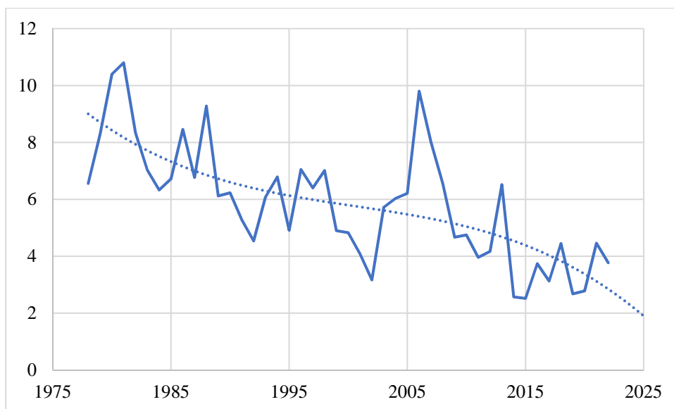
Рис. 6. Динамика среднегодовых расходов воды ( Q , м 3 /с) р. Ворсклы (пост Козинка) за 1978–2022 гг. (прогноз до 2025 года)
