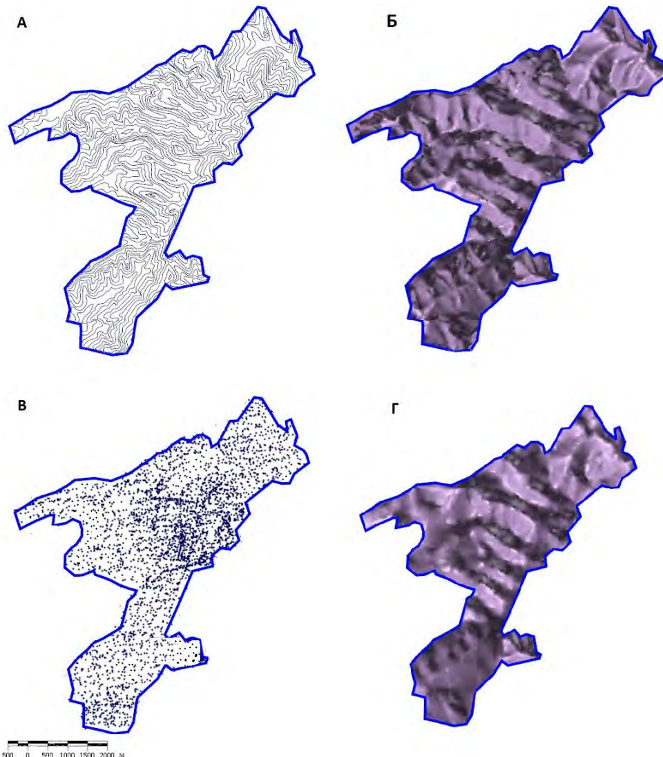
Рис. 1. А) Изолинии с топографической карты; Б) «историческая» ЦМР; В) Облако точек по данным SRTM; Г) ЦМР, построенная по данным SRTM
