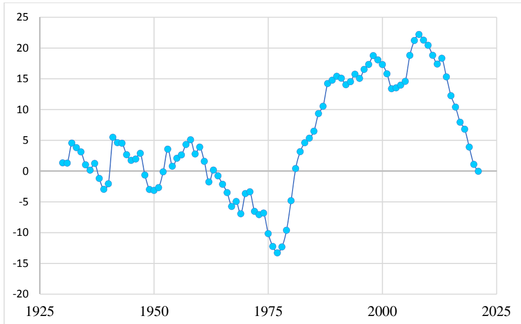
Рис. 4. Разностная интегральная кривая среднегодовых расходов ( Q , \text{m}^3/\text{с} ) р. Ворсклы (пост Козинка) за период 1930–2022 гг. Fig. 4. Difference integral curve of average annual flow rates ( Q , \text{m}^3/\text{s} ) Vorskla River (Kozinka post) for the period 1930–2022
