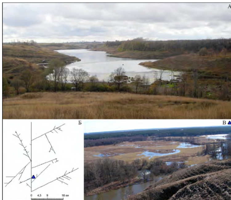
Рис. 1. Зона истока р. Ворсклы у с. Покровка Ивнянского р-на (А); граф гидрографической сети в границах Борисовского р-на (Б); вид на долину реки с детинца Хотмыжского городища (В)
