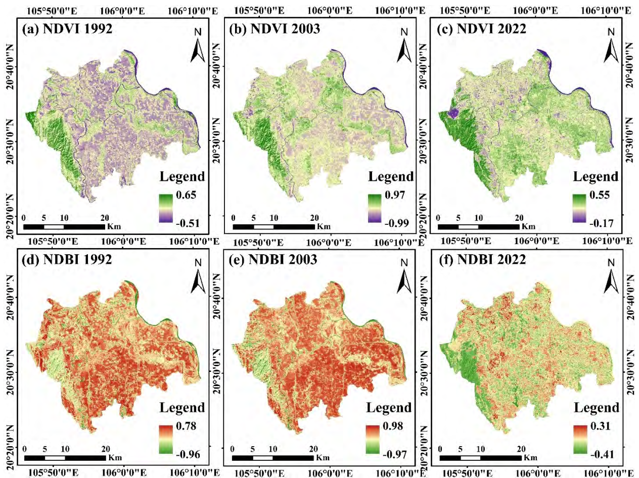
Fig. 5. NDVI and NDBI maps for Ha Nam province in 1992, 2003, and 2022 Рис. 5. Карты NDVI и NDBI провинции Ханам в 1992, 2003 и 2022 годах
