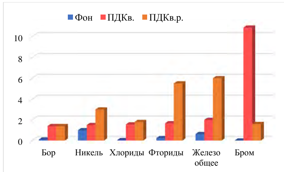
Рис. 7. Превышения предельно допустимых концентраций для питьевого и культурно-бытового водопользования, согласно СанПиН 1.2.3685-21 (ПДКв.) и рыбохозяйственного водопользования (ПДКв.р.) основных загрязняющих веществ в Крапивненском вдхр. и в р. Ворскле у п. Яковлево (Фон) по данным за 2019–2021 гг.
