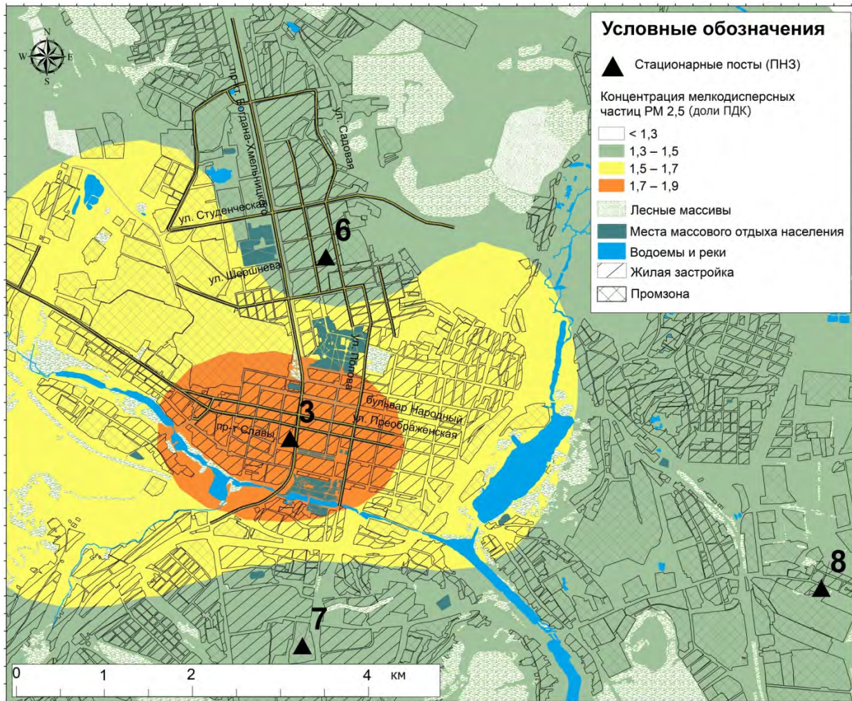
Рис. 2. Распределение среднегодовых концентраций PM2.5 в атмосферном воздухе Белгорода
