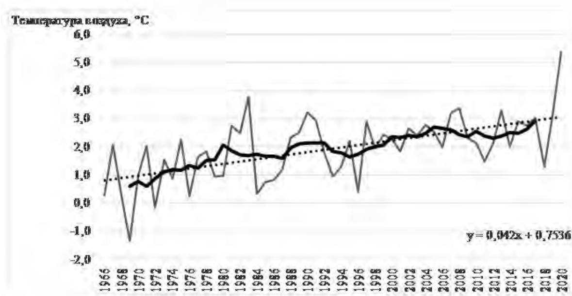
Рис. 1. Многолетний ход средней годовой температуры воздуха за 1966–2020 гг. на метеостанции Петропавловск
