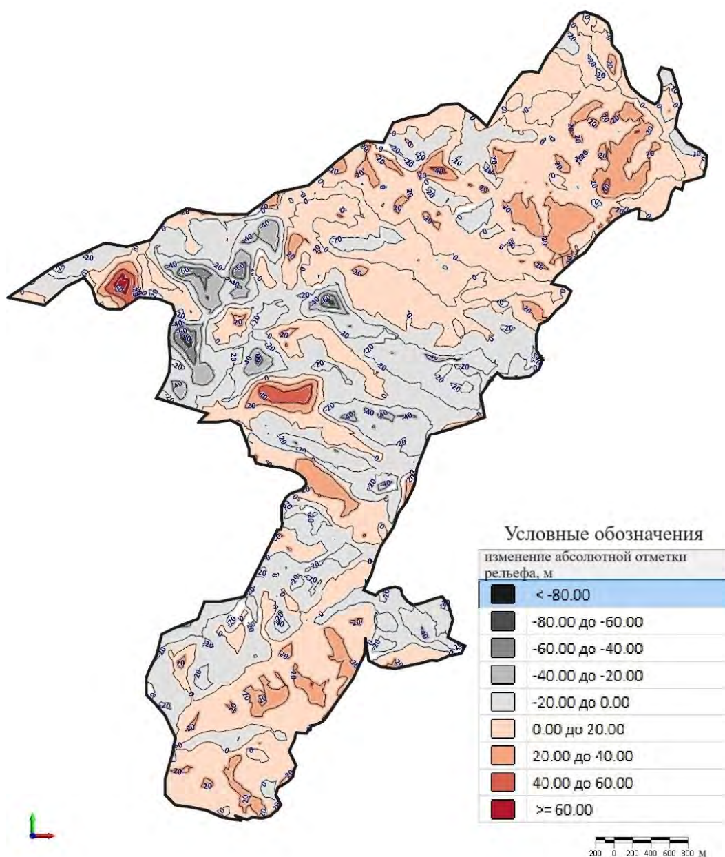
Рис. 2. Карта техногенной трансформации рельефа территории углеразреза «Распадский» Fig. 2. Map of anthropogenic transformation of relief on the territory of Raspadsky coal strip mine
