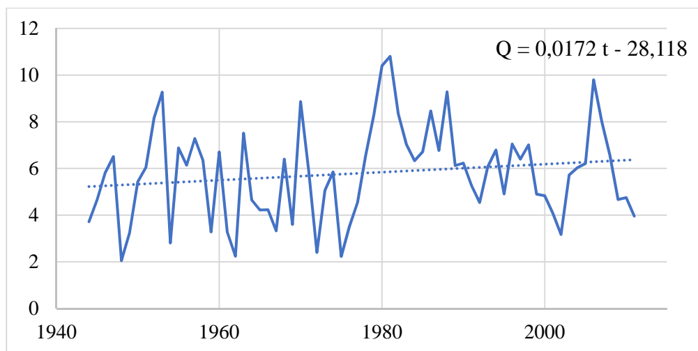
Рис. 2. Среднегодовые расходы воды (Q, м 3 /с) р. Ворсклы (пост Козинка) за 1944–2011 гг. [Лисецкий и др., 2015, с. 106, рис. 3.2]
