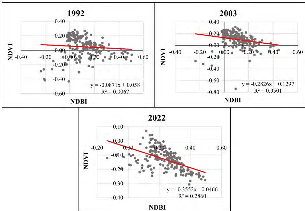
Fig. 6. Regression analyses between NDVI and NDBI in Ha Nam province Рис. 6. Регрессионный анализ между NDVI и NDBI в провинции Ханам
