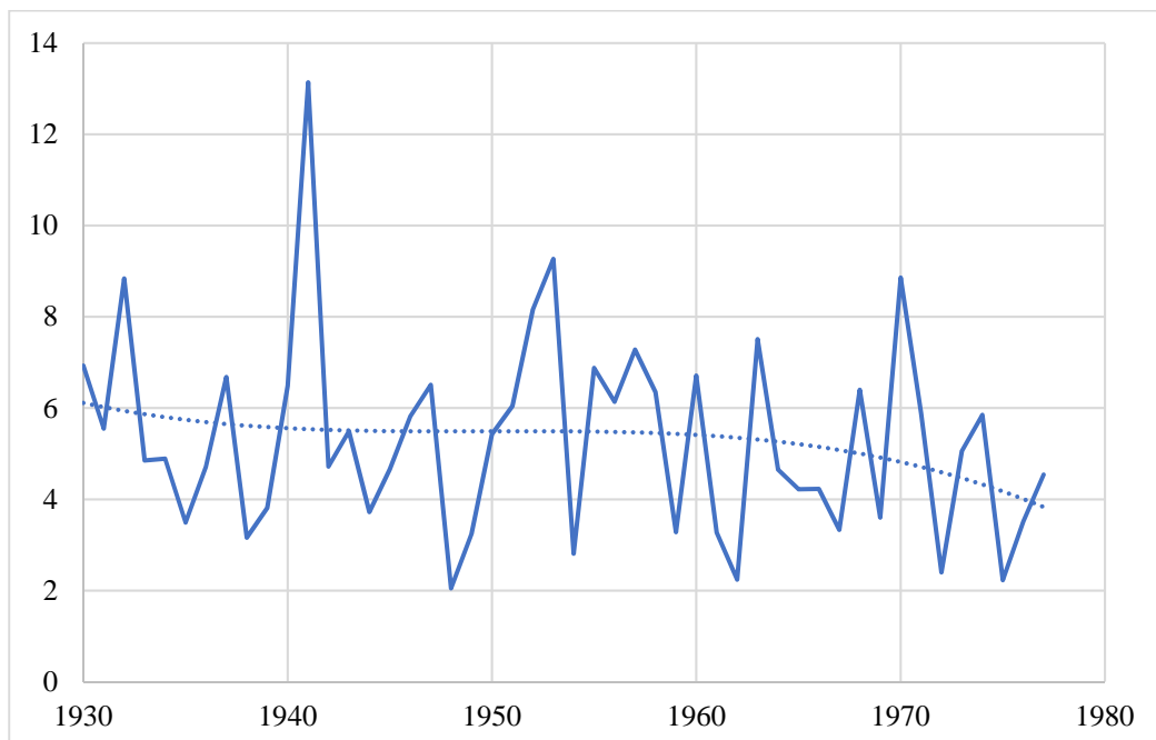
Рис. 5. Динамика среднегодовых расходов воды ( Q , \text{m}^3/\text{с} ) р. Ворсклы (пост Козинка) за 1930–1977 гг. Fig. 5. Dynamics of average annual water flow ( Q , \text{m}^3/\text{s} ) Vorskla River (Kozinka post) for 1930–1977
